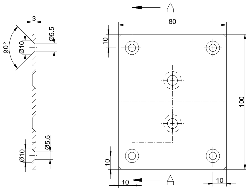
Schnitt A-A
