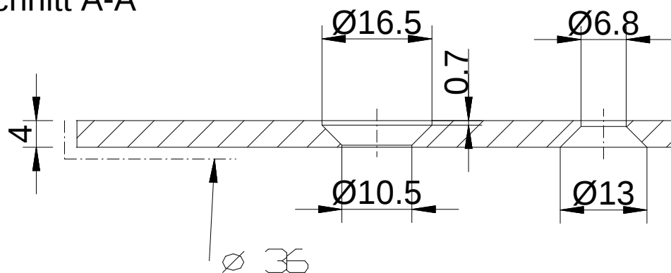
Schnitt A-A
