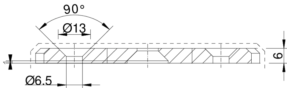
Schnitt A-A
