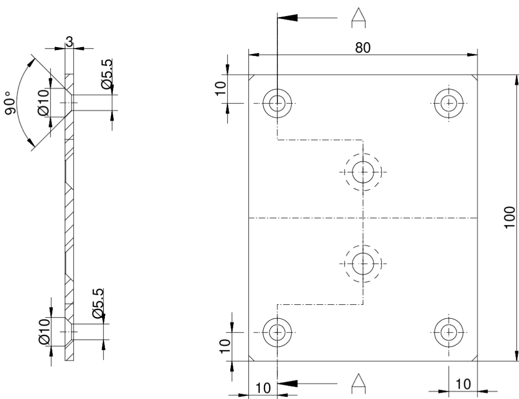
Schnitt A-A
