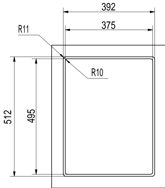
Flächenbündiger Einbau
