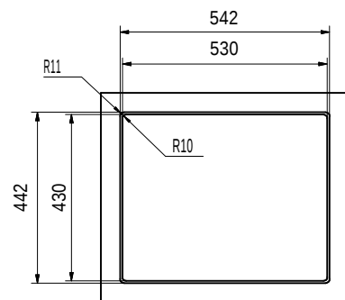
Detail 1 : 2
