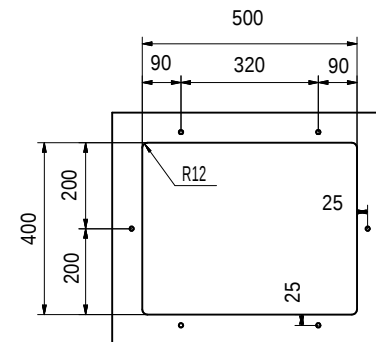
Unterbauspüle Befestigungsbohrungen an der Unterseite 6 Bohrungslocher ø 10 mm, Tiefe 15 mm
