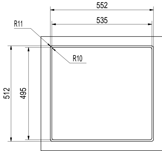
Flächenbündiger Einbau
