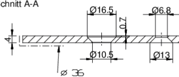
Schnitt A-A
