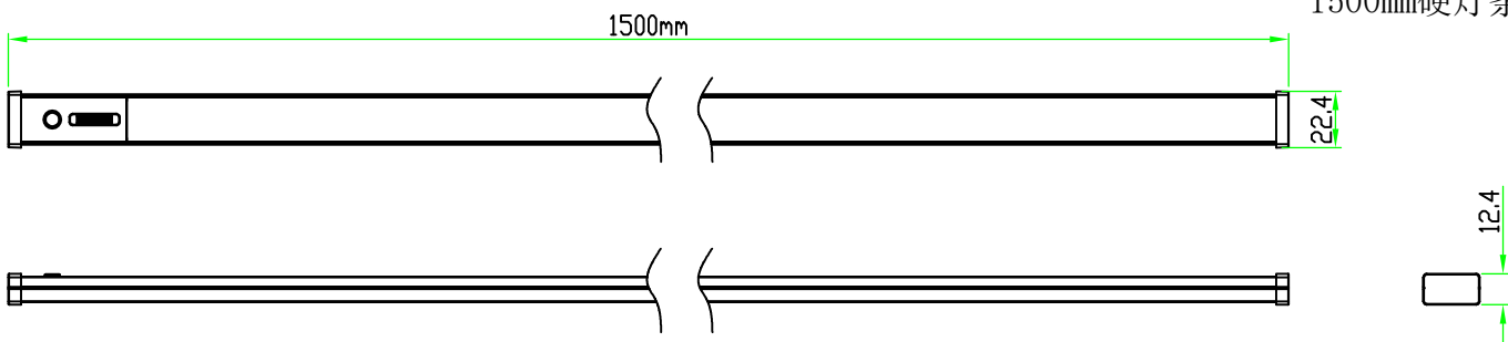
1500mm硬灯条
