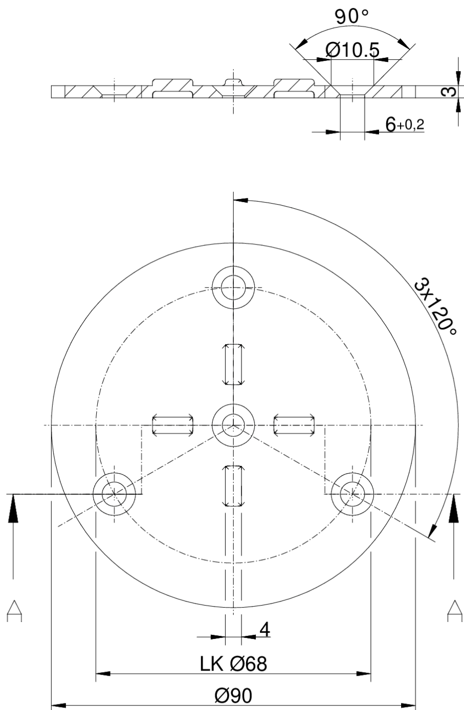
Schnitt A-A
