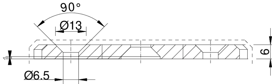
Schnitt A-A
