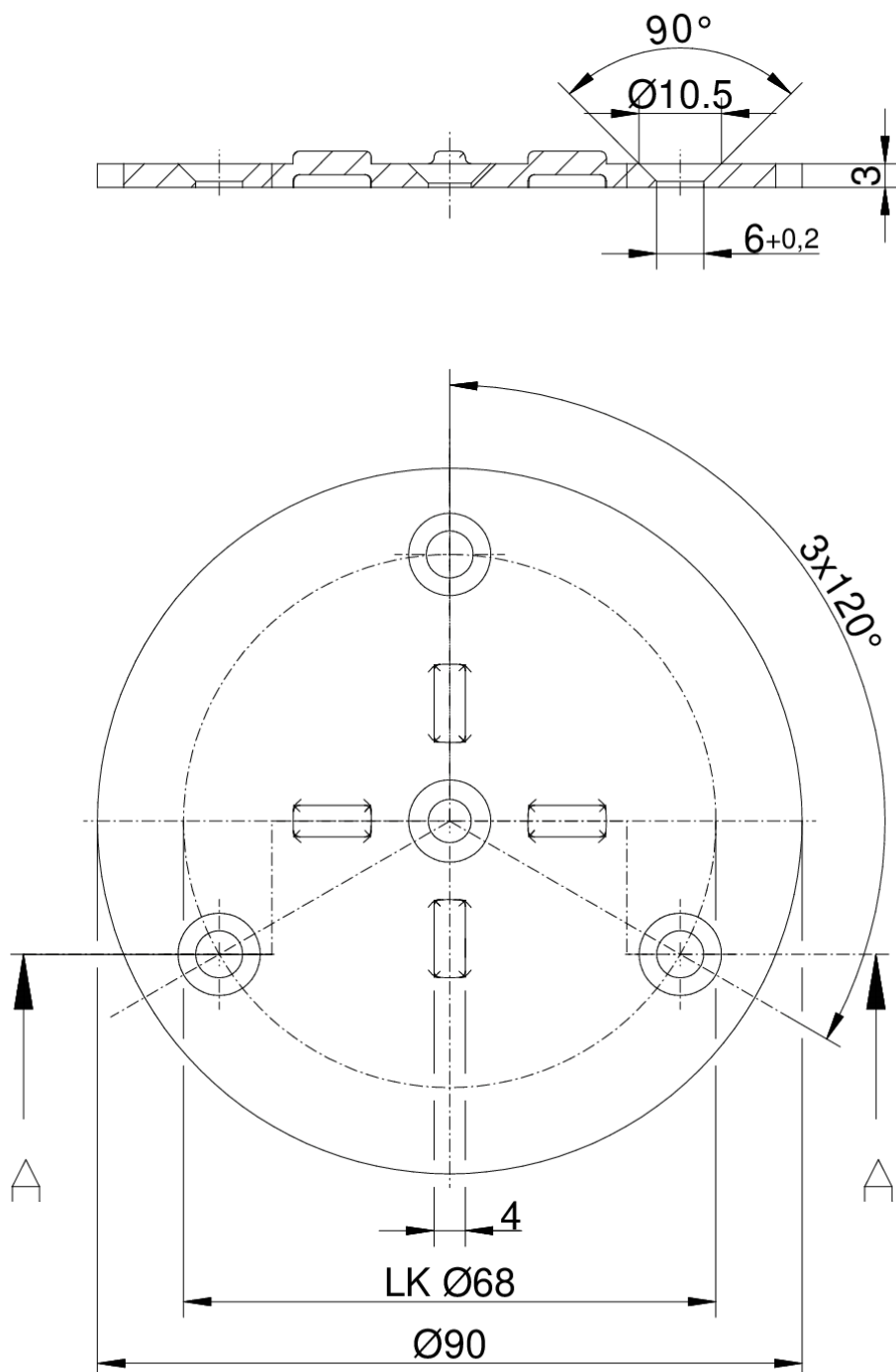
Schnitt A-A
