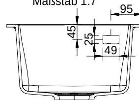
Schnittansicht A-A Maßstab 1:7
