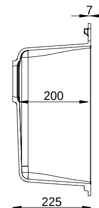
Schnittansicht B-B Maßstab 1:7
