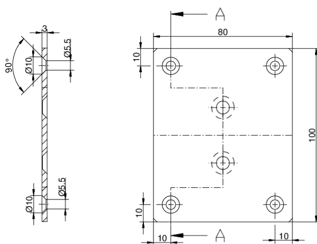
Schnitt A-A
